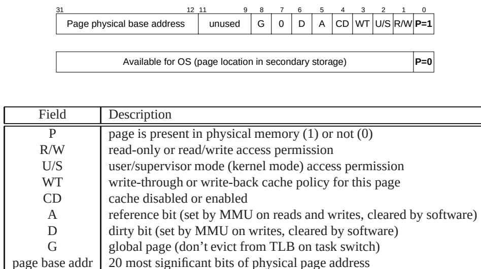
(b) Page Table Entry (PTE).
